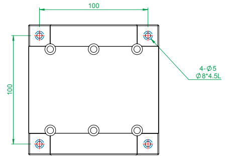
MX(Y)120-A系列 底座安裝孔尺寸
