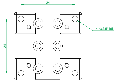
MX(Y)L30-A系列 底座安裝孔尺寸
